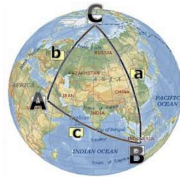
Gambar 1: Ilustrasi Segitiga Bola 15
